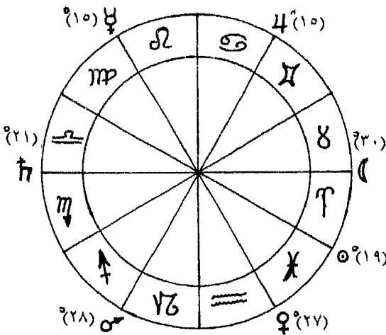
شكل (١٦) : أماكن إشراق وهبوط الكواكب
